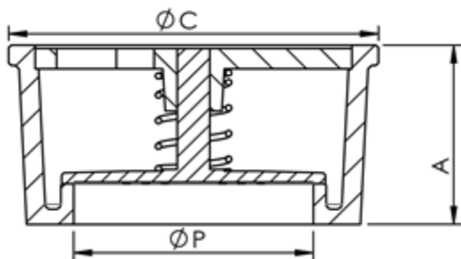
Габаритные и присоединительные размеры обратных затворов.
