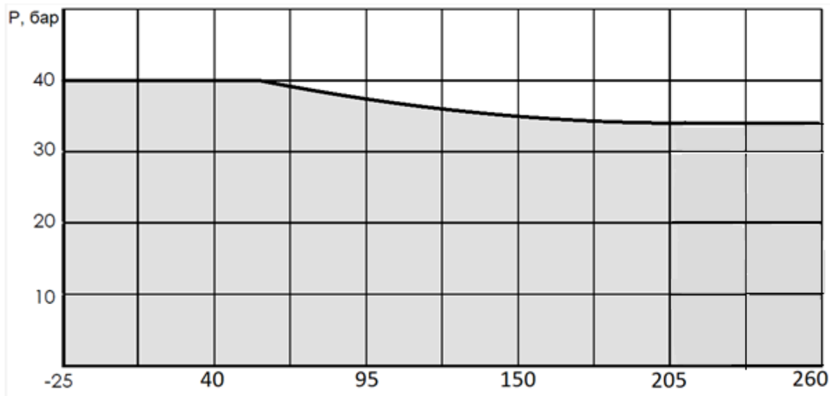
Диаграмма Температура-Давление
